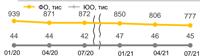
Кількість клієнтів
